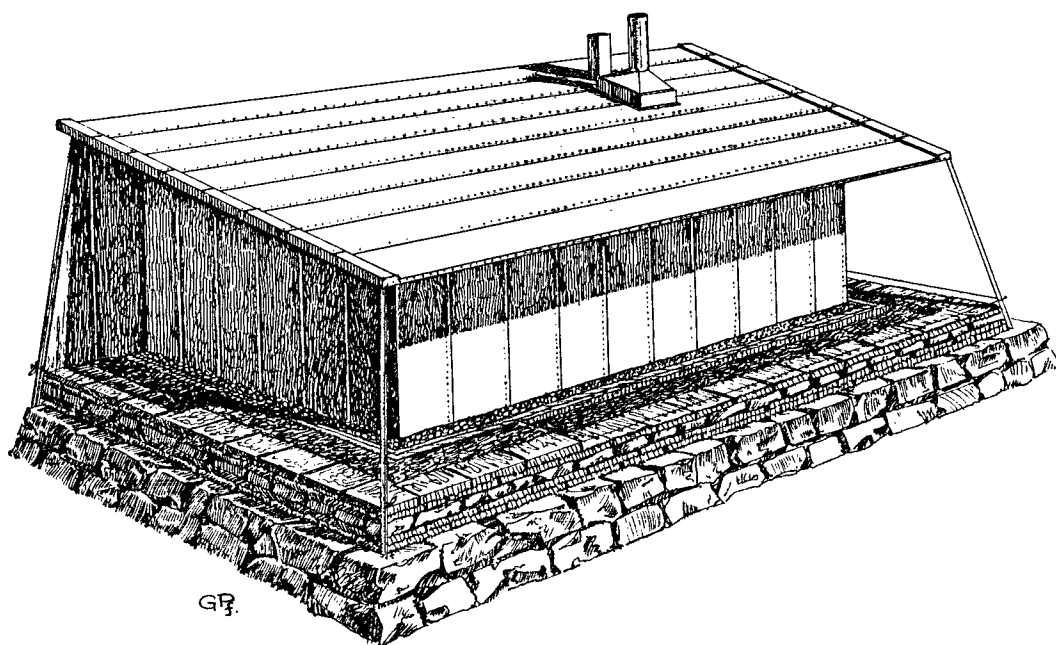
Fig. 3. Princippet for murens opførelse.
