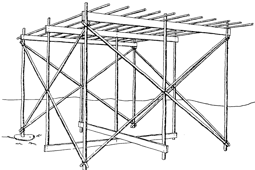
Fig. 1. Stillads til tørring af hundefoder til vinterbrug. Stilladset er beregnet til at bære 2.000 kg og til at stå ubelastet eller belastet for store stormstyrker, selvom det opsættes på bar klippe.
