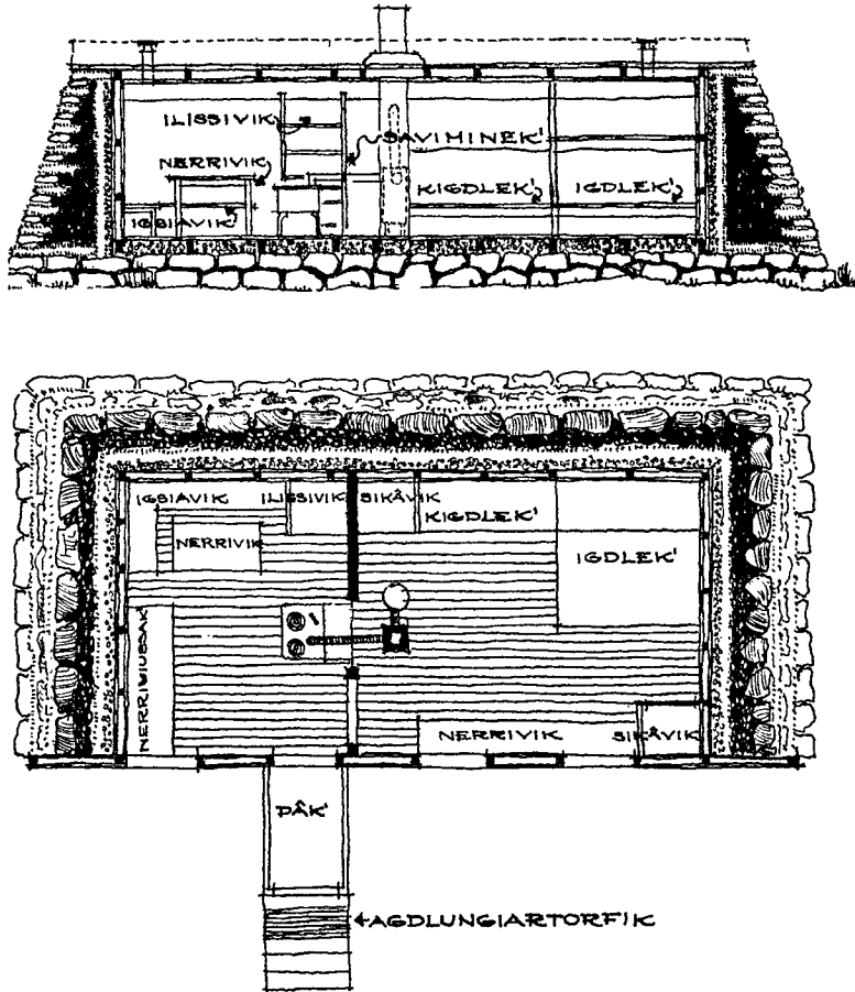
Fig. 4. Tørvevurshus med spisekøkken og med stue med faste skabe, fast bord samt tre køjer for børnene og briks for forældrene. Komfuret bidrager til stuens opvarmning, idet den lodrette jernplade bag dette har ventilation ved loft og gulv.
