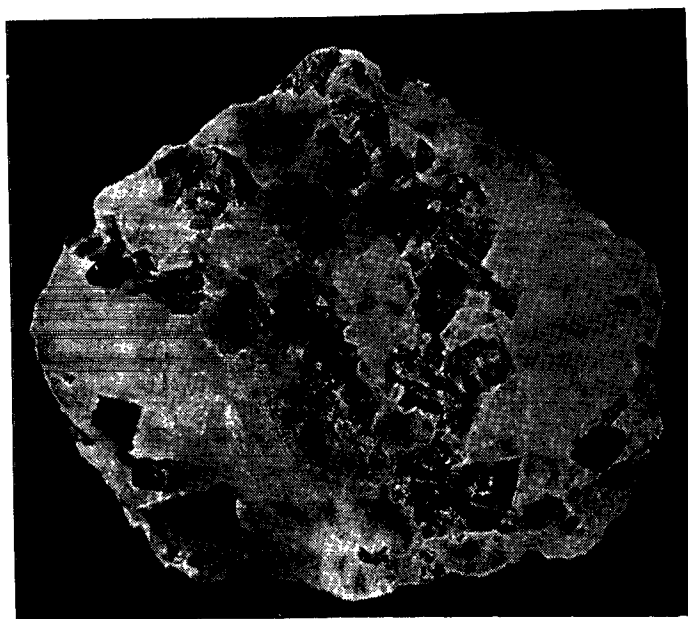
RÅKRYOLIT FRA IVIĞTUT
