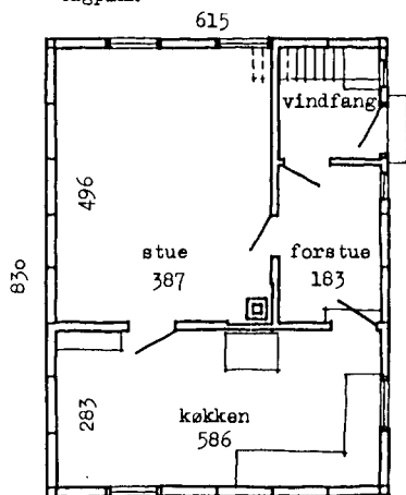
stueplan
